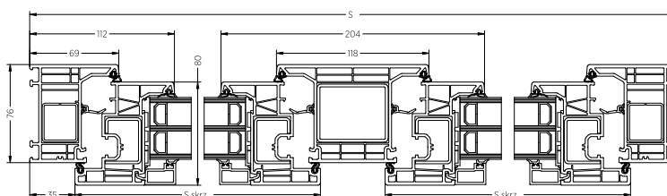
Przekrój poziomy skrzydło okienne, słupek szeroki
