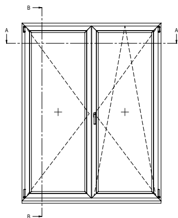
Okno dwuskrzydłowe z ruchomym słupkiem w systemie Softline 82 Widok od wewnątrz
