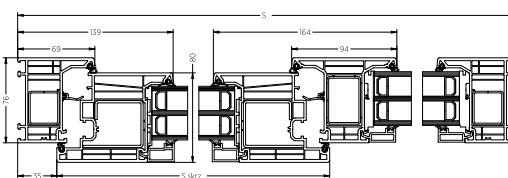
Skrzydło szerokie, słupek standard
