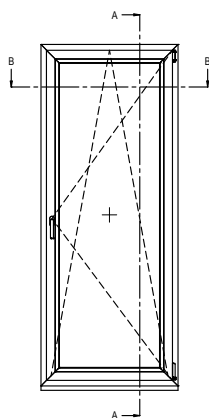
Okno jednoskrzydłowe rozwierno-uchylne w systemie Scotline 82 Widok od wewnątrz
