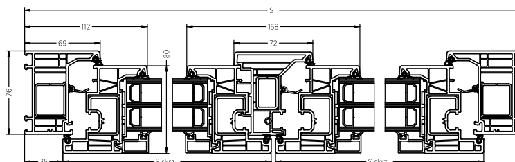
Przekrój poziomy
