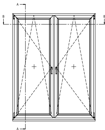
Okno dwuskrzydłowe ze słupkiem stałym w systemie Softline 82 Widok od wewnątrz
