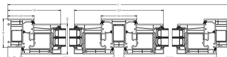
Przekrój poziomy skrzydło szerokie, słupek standard
