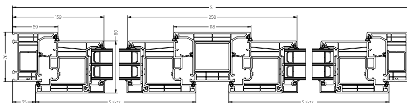
Przekrój poziomy, skrzydło szerokie, słupek szeroki
