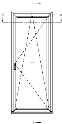
Okno jednoskrzydłowe rozwierno-uchylne w systemie Sofiline 82 z niskim progiem Widok od wewnątrz
