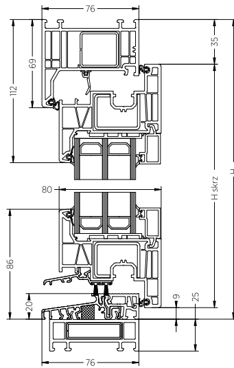
Przekrój pionowy
